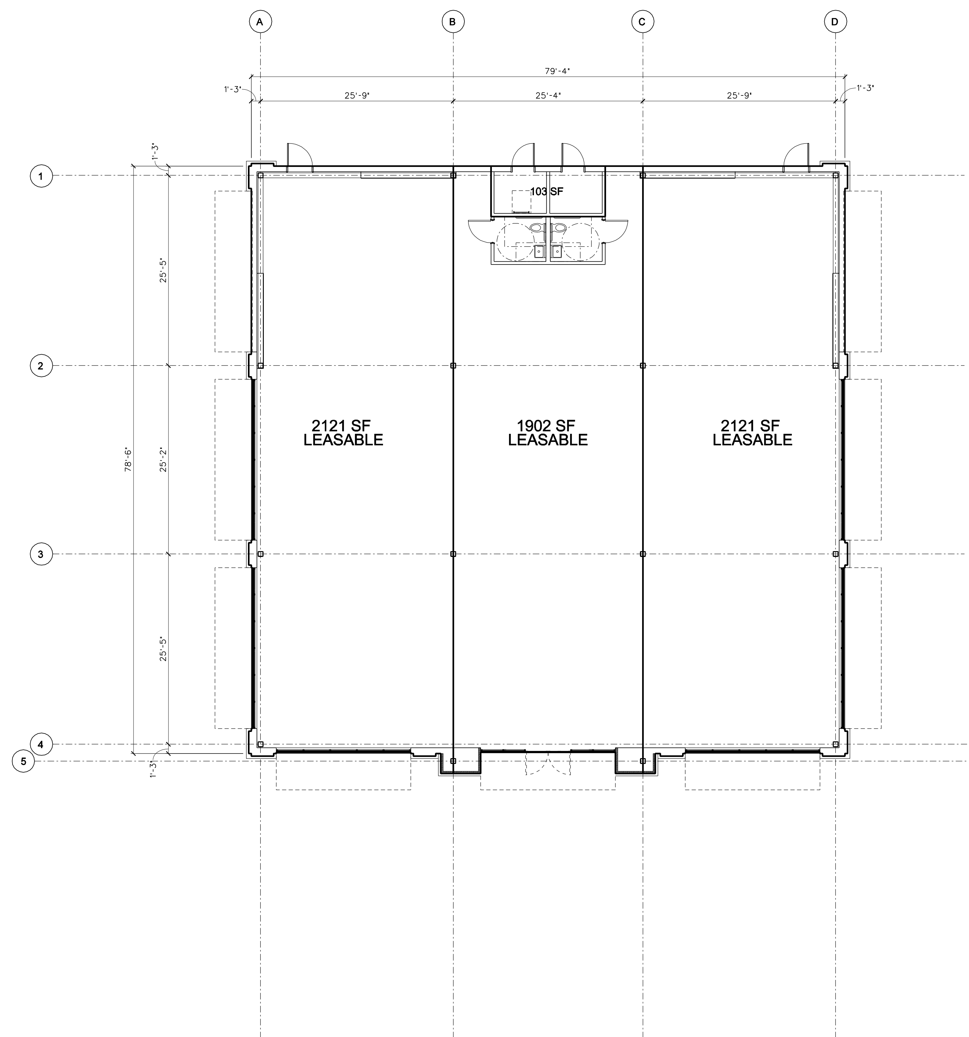
A5 LEASING PLAN SCALE: 1/8" = 1'-0"
